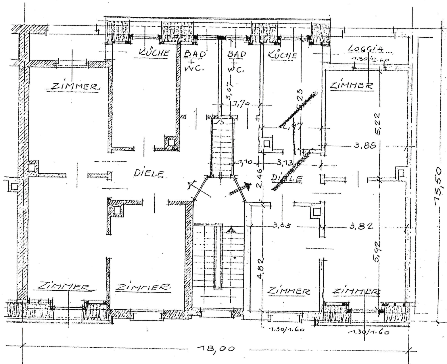
GRUNDRISS: III. OBERGESCHOSS - RECHTS DACH - GESCHOSS
